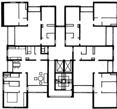
Figure 9. Typical floorplan of housing unit in Märkisches Viertel, Berlin. O. M. Ungers (1962–67). Courtesy of the Ungers Archiv für Architektur wissenschaft.
