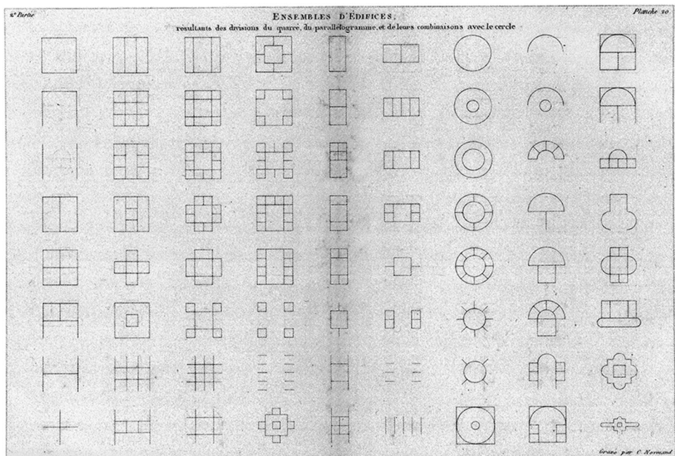
Figure 10. 'Plate 20, Ensemble d'édifices, résultants de divisions du carré, du parallélogramme et de leurs combinaisons avec le cercle' [Building Ensembles, Resulting from the Divisions of the Square, the Parallelogram and Their Combinations with the Circle], in Jean-Nicolas-Louis Durand, Précis des leçons d'architecture données à l'École Royale Polytechnique , vol 1 (Paris: the author, 1802).
